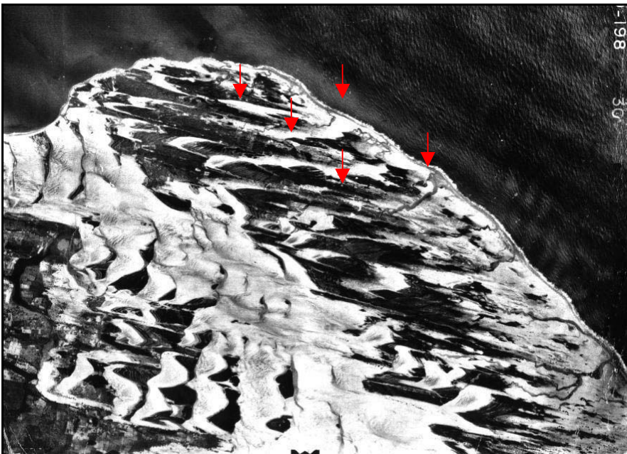
Figura 2 – Fotografia aérea de 1969, mostrando a ocorrência de dunas parabólicas associadas ao fenômeno La Niña. Fonte: DNPM (1969).
