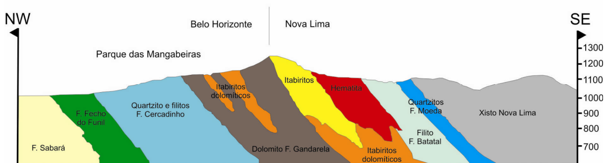
Figura 4 – Secção geológica Fonte: Adaptado de Grandchamp, 2003.
