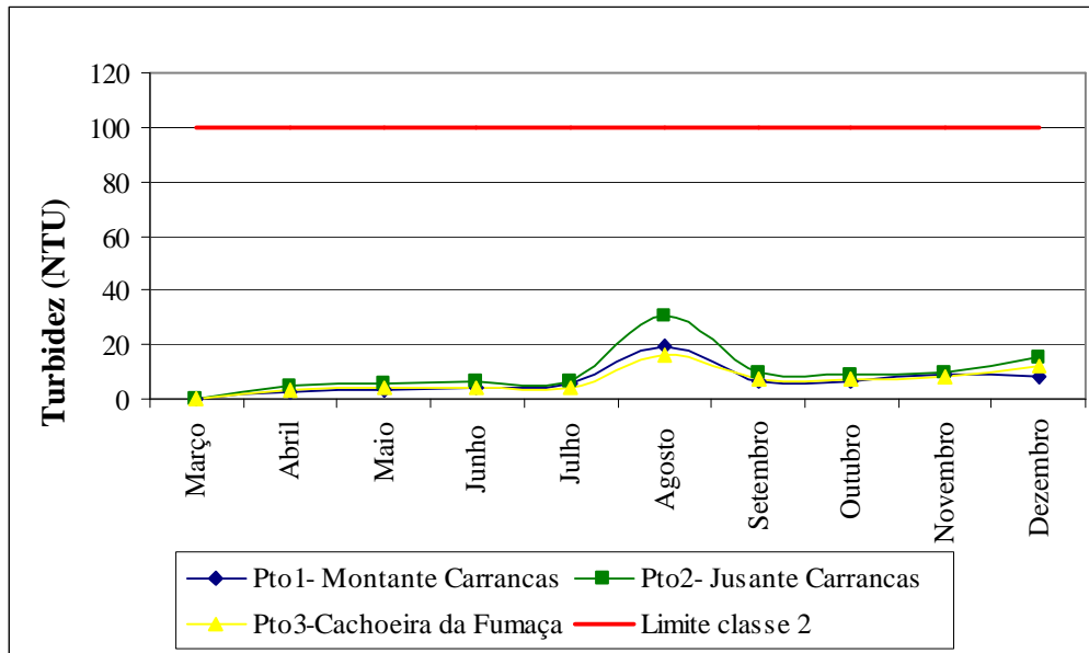
Figura 4 – Monitoramento de turbidez no Ribeirão de Carrancas/MG
