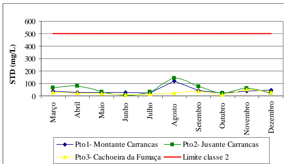
Figura 3 – Monitoramento de sólidos totais dissolvidos (STD) no Ribeirão de Carrancas/MG.
