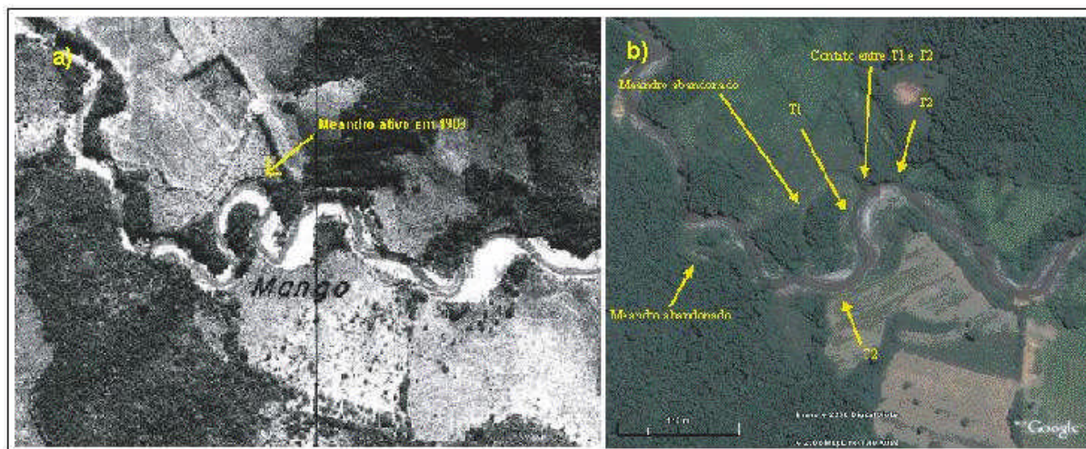
Figura 4 – Migração lateral da calha do Ribeirão do Mango: a) ortofoto de 1989 - destaque para meandramento ativo; b) Imagem Google 2008 - destaque para meandro abandonado e T1
