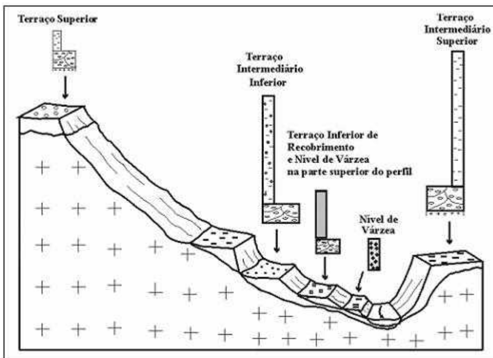
Figura 2 – Perfil transversal do vale do Ribeirão do Mango e respectivos níveis deposicionais.
