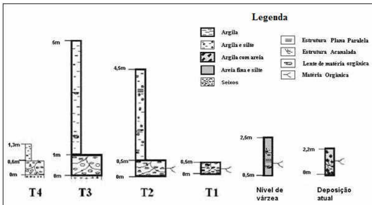
Figura 3 – Perfis síntese dos depósitos aluviais analisados.
