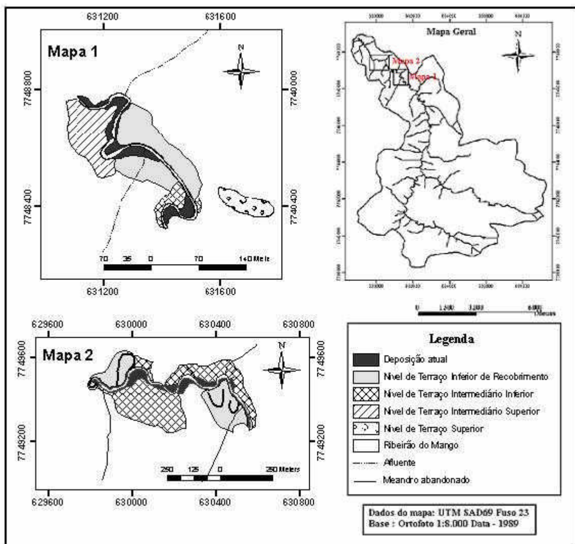
Figura 5 – Arranjo espacial dos níveis aluviais em trechos do vale do baixo ribeirão do Mango
